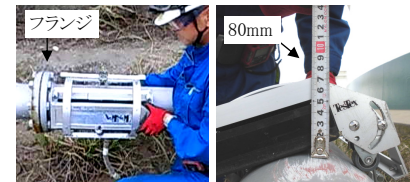
フランジ近傍の探傷 (未探傷範囲なし)
